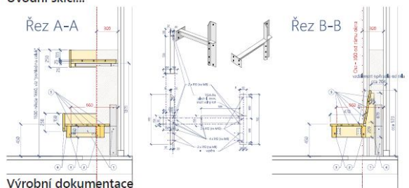
Výrobní dokumentace
